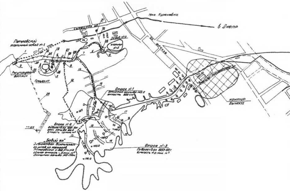
Рис. 16. План реконструкции систем водоснабжения и гидротранспорта на карьерах Петровских кирпичных заводов. 1957 г.
