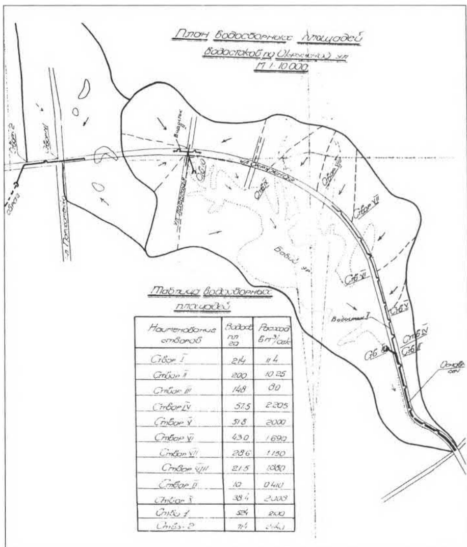
Рис. 18. План водосборных площадей водосток по Окружной ул. 1961 г.
