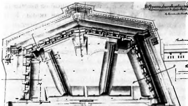
Чертеж укрепления «Граф Берг».
